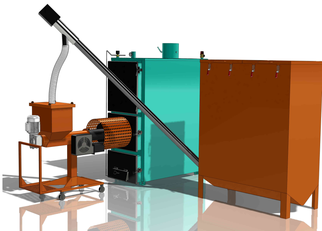
EE 100 kW katls ar granulu degļa pieslēgumu no katla priekšpusēs
