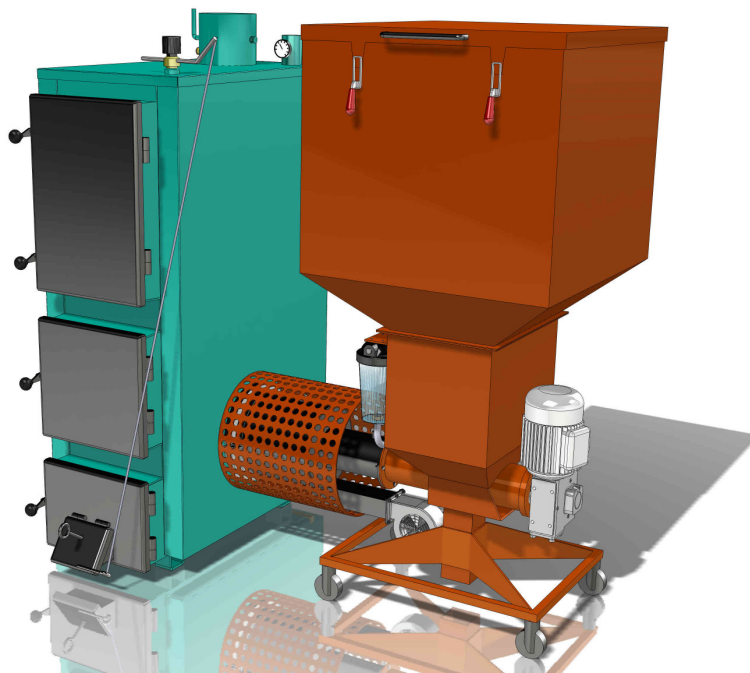
Cietā kurināmā katls un granulu deglis ar 150 L bunkuru
