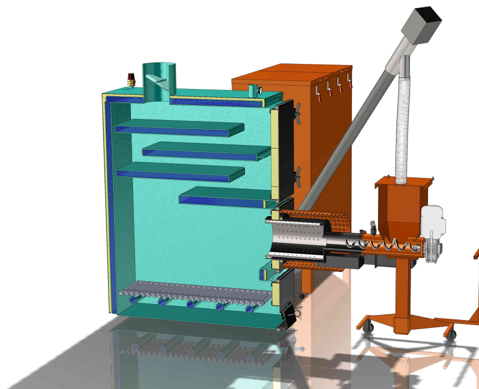
80-150 kW katls ar granulu degli. Šķērsgriezums
