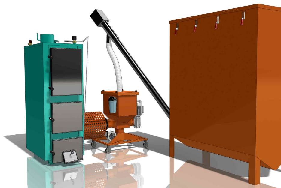
EE 40 kW katls. Kompaktais granulu deglis ar papildus transportieri
