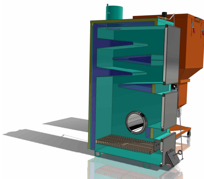
25-50 kW katls ar granulu degli. Šķērsgriezums
